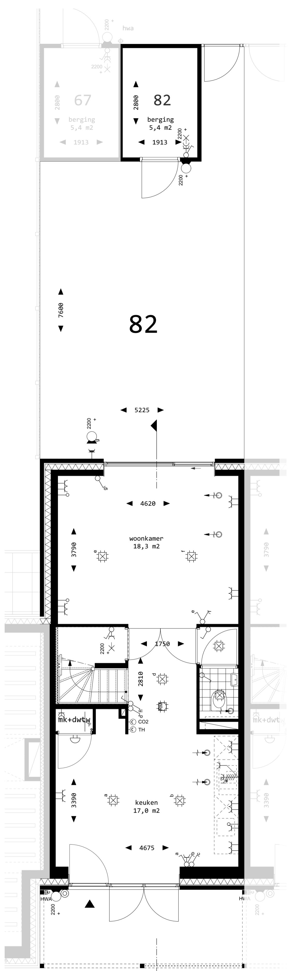
begane grond
