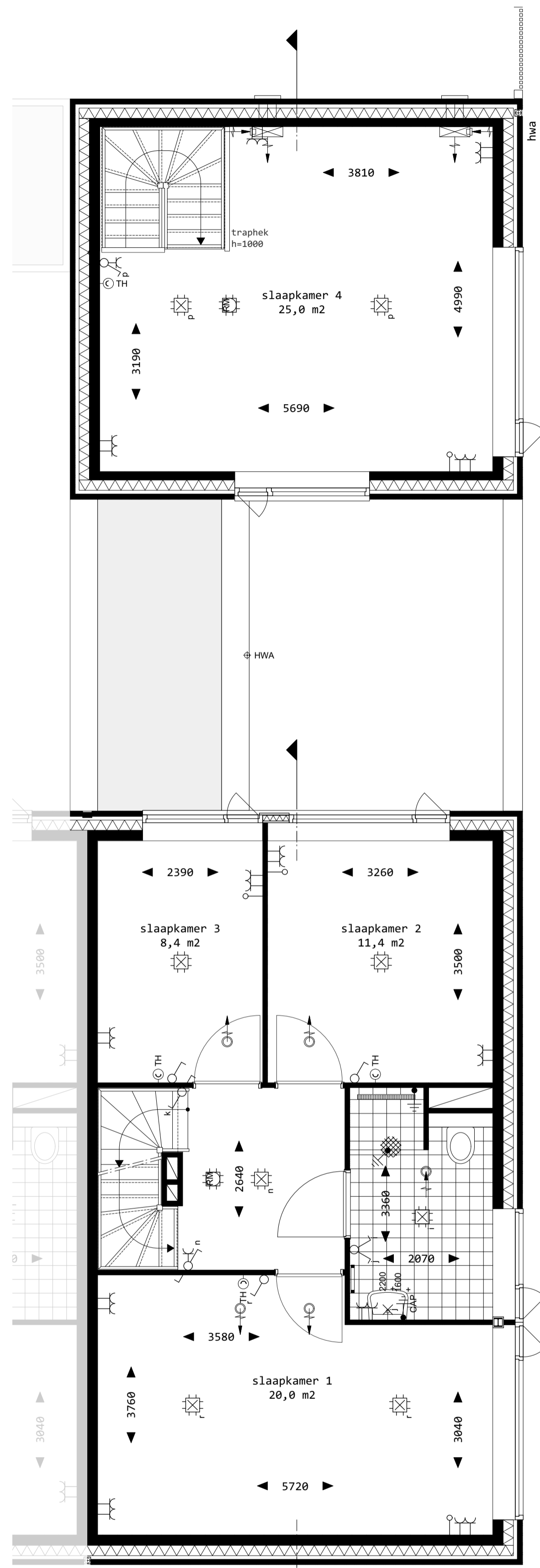
1e verdieping
