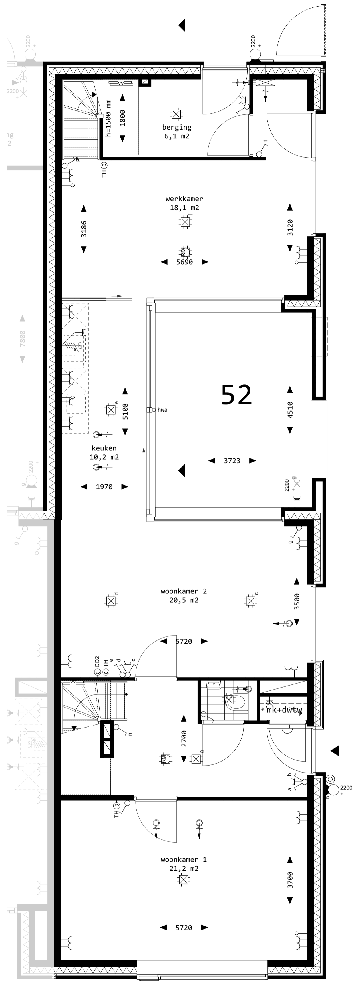
begane grond
