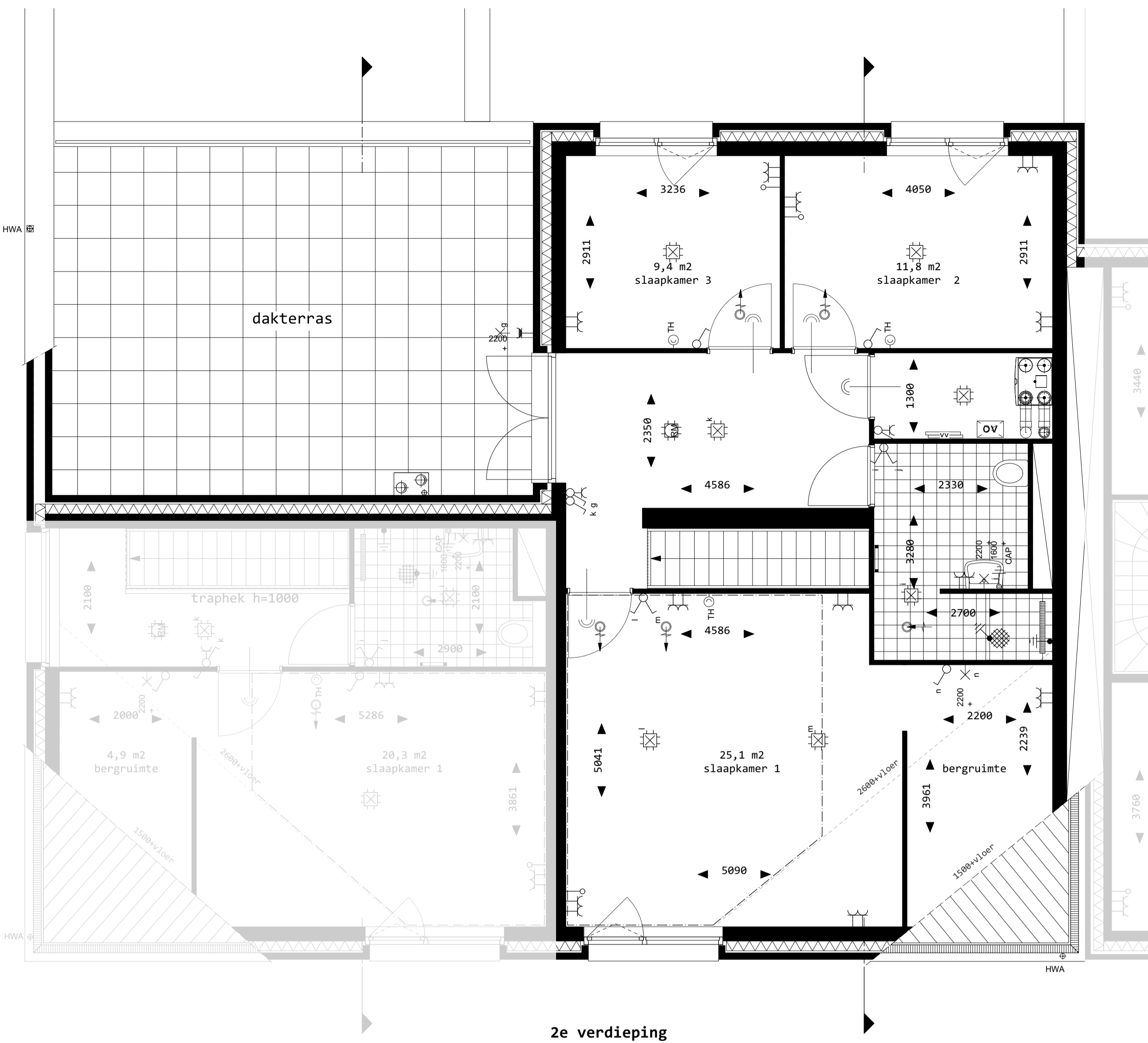
2e verdieping
