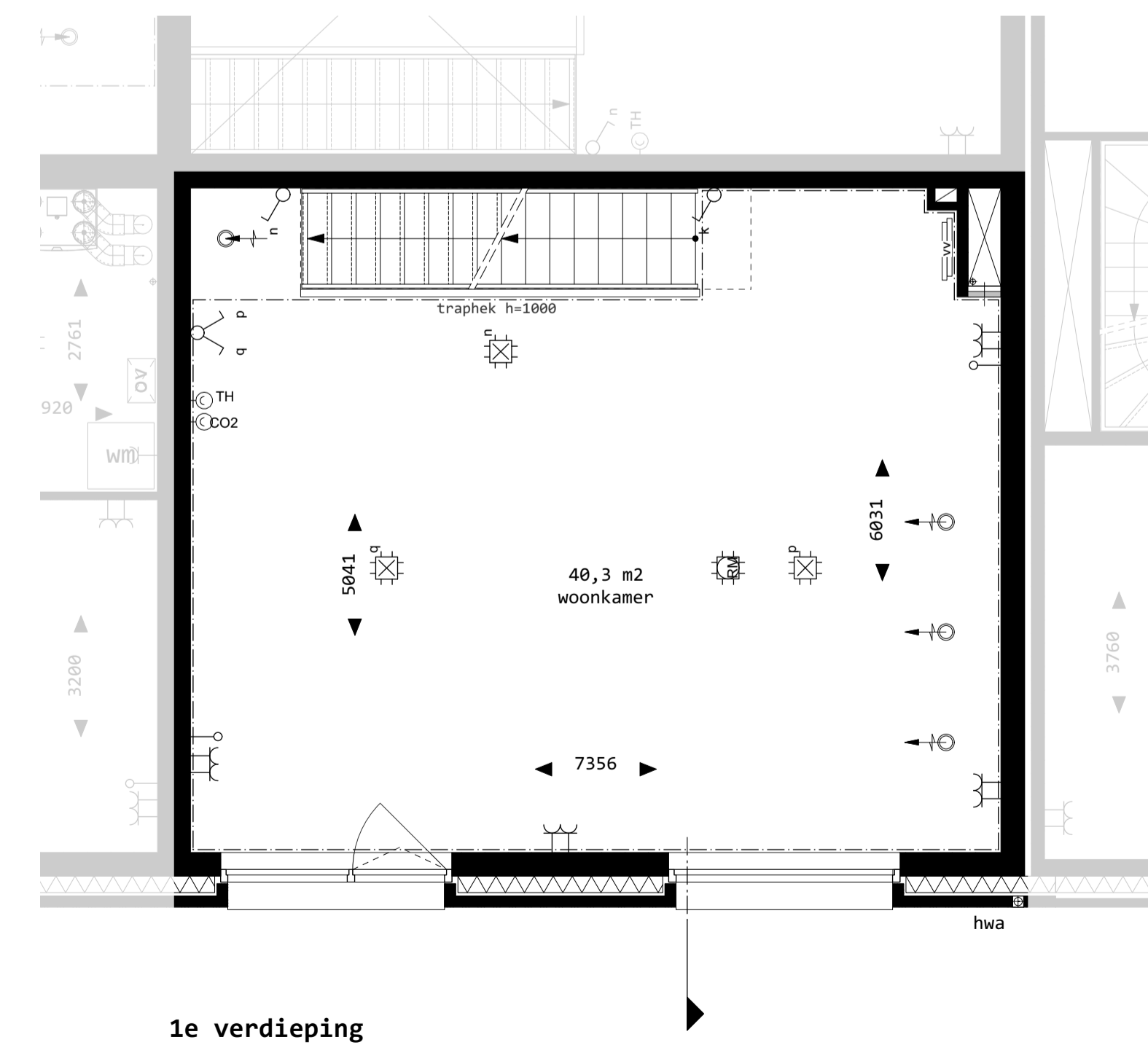
1e verdieping
