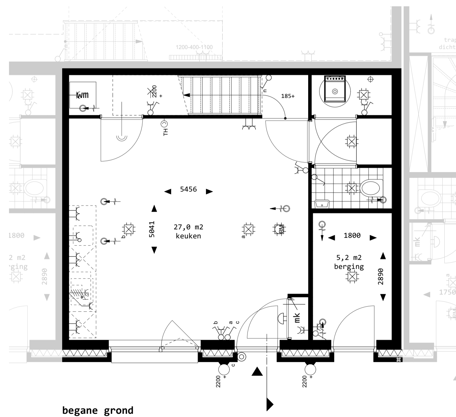
begane grond
